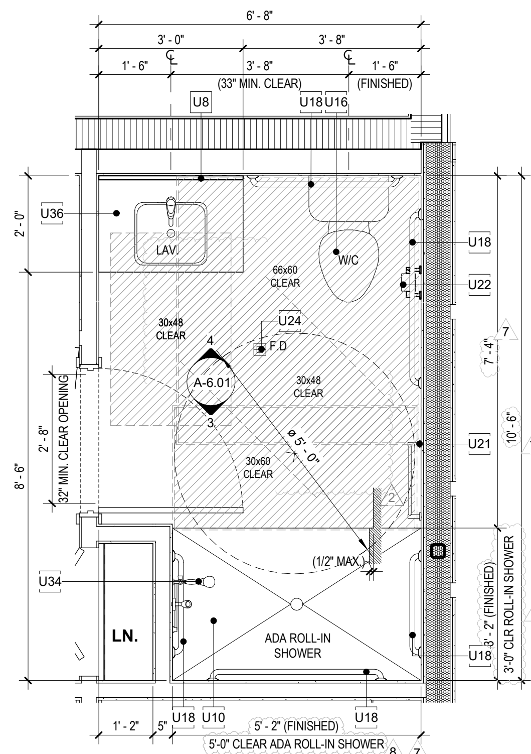
UNIT A2 FA BATHROOM PLAN SCALE: 1/2" = 1'-0"
